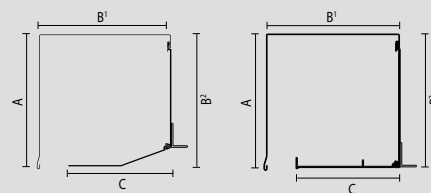
T-UP Kastengrößen in mm
