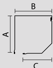
T-5E Kastengrößen in mm
